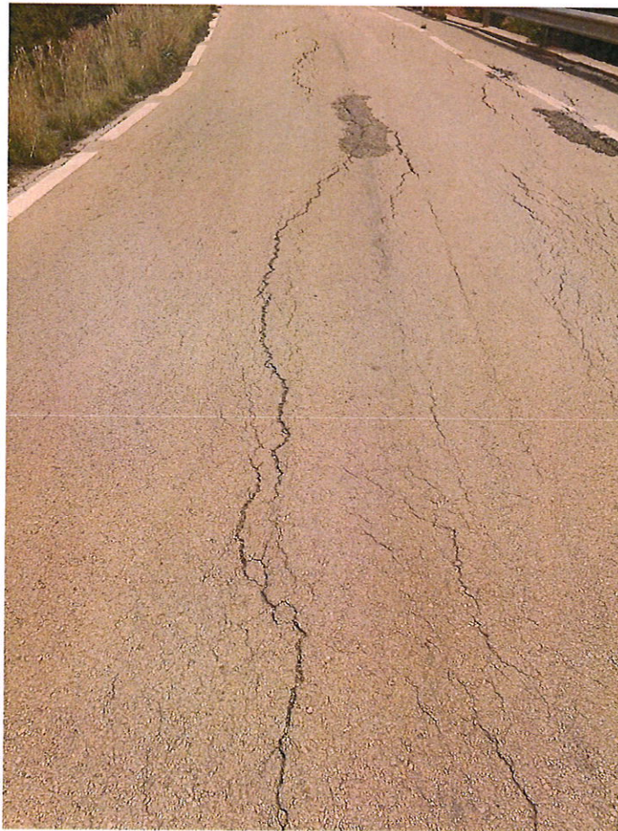
Problemas en el firme de la RM-320
